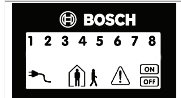
Figura 2: Pantalla del teclado LCD de ocho zonas ICP-CP508LW
